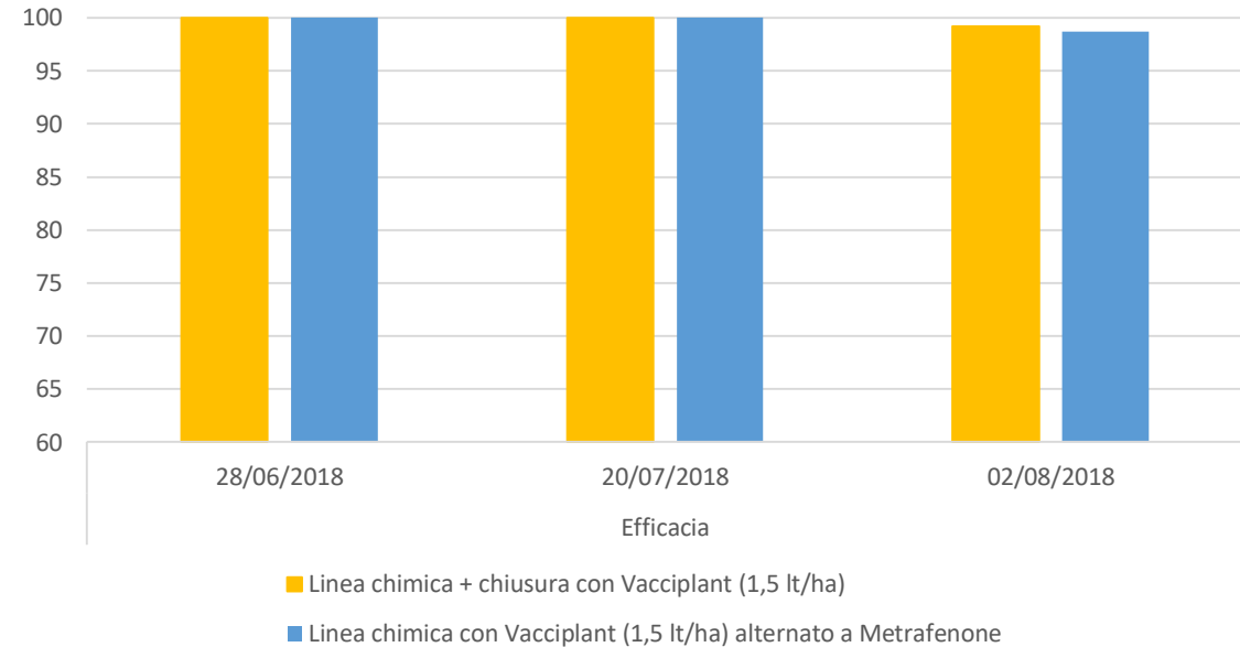
Efficacia Abbott %
